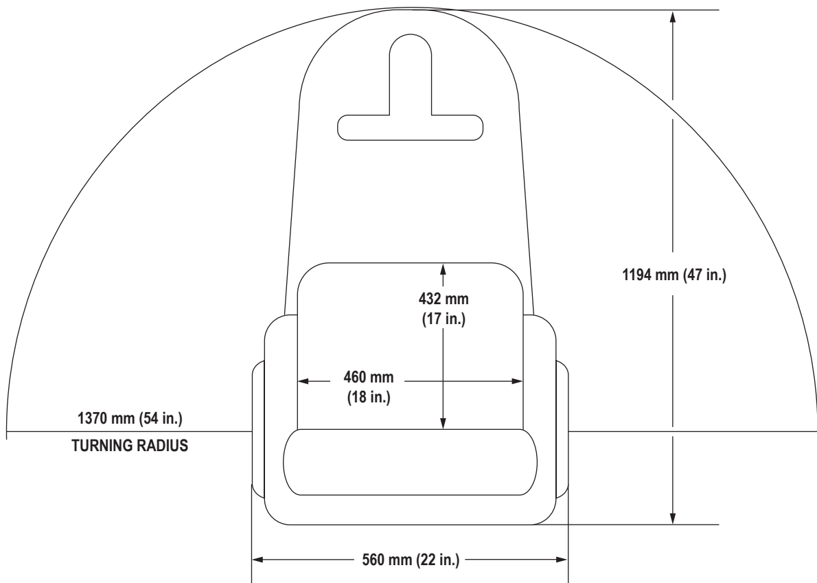
Colt Plus (SC710) Dimensions
