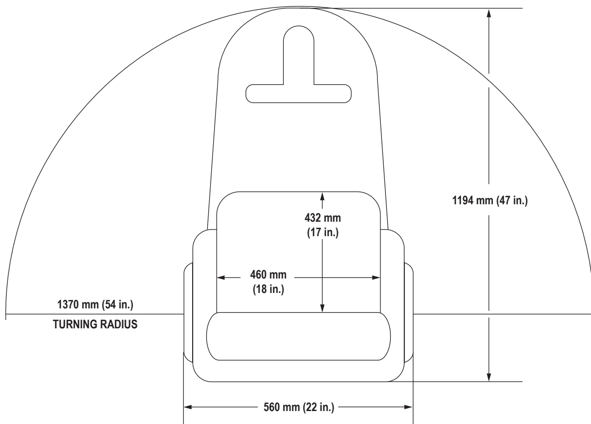
Colt Plus (SC710) Dimensions
